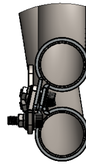
詳細図 C スケール 2 : 5
