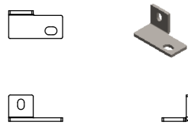
YML258 フロントバンク
