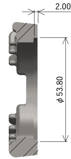
断面図 B-B
