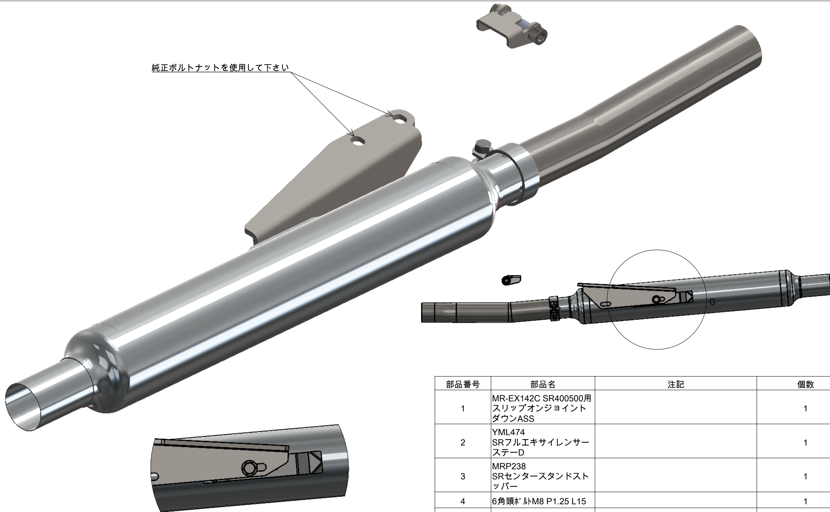
詳細図 G スケール 2 : 5
