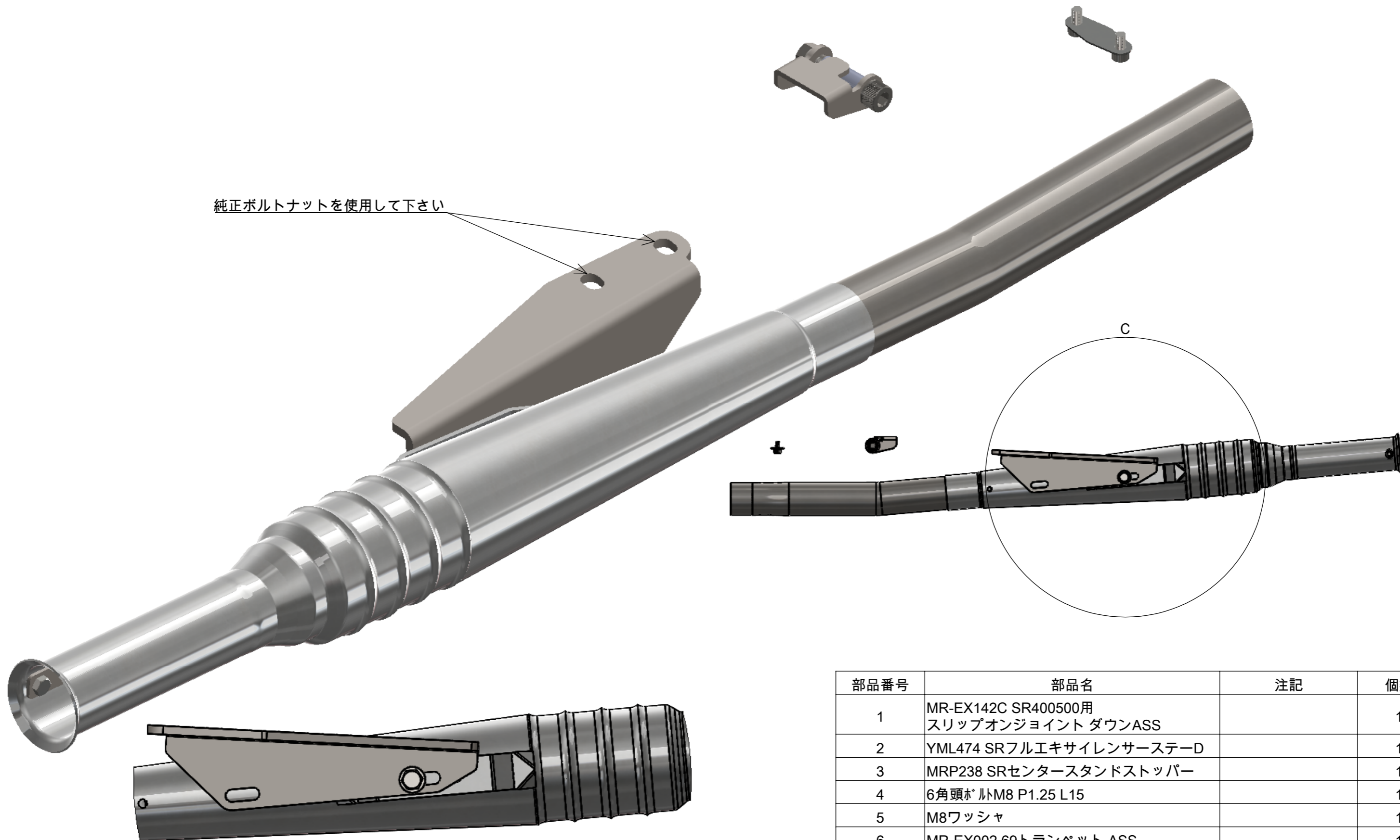
詳細図 C スケール 2:5
