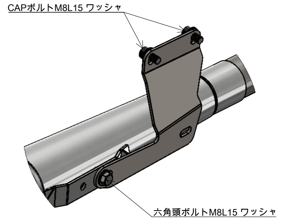
詳細図 B スケール 2 : 5
