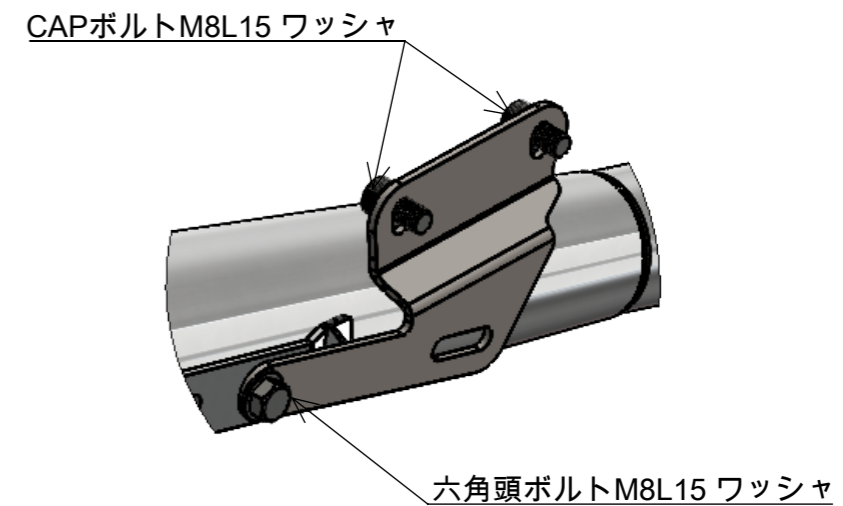
詳細図 F スケール 2 : 5
