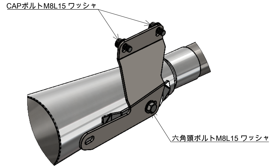
詳細図 B スケール 2 : 5
