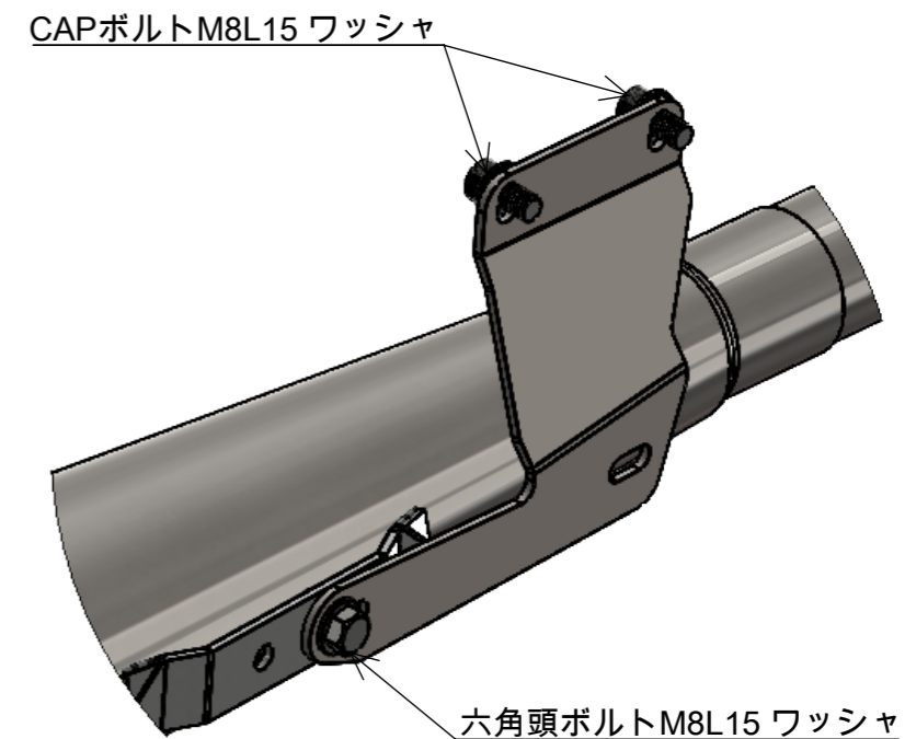
詳細図 B スケール 2 : 5
